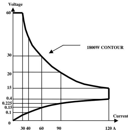
圖 1-2 3351F 高功率電子負載功率曲線圖
