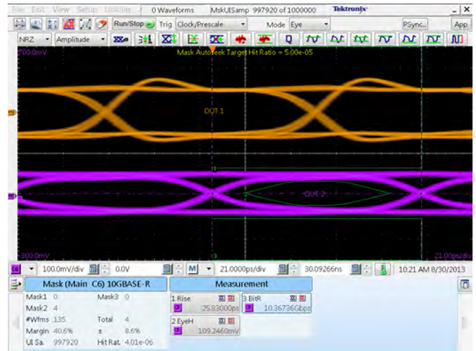
光接口眼图测试
