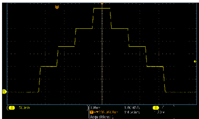
图7B 使用清单模式自动设置输出电压。通过清单建立的电压如7A所示。
