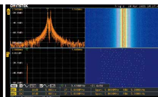
双通道频谱分析仪+光谱图
