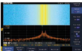
频谱分析仪+光谱图
