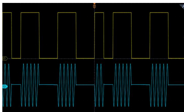
脉冲调制输出实测
