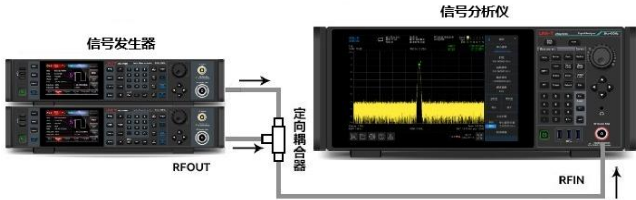
图 3-4：获取两路信号的仪器设置
