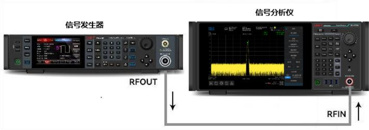
图 3-10：获取单一信号的仪器设置
