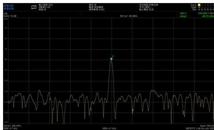
图 3-12: 在 0dB 衰减下测量小信号
