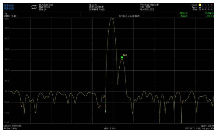
图 3-9：大信号中分辨出的小信号
