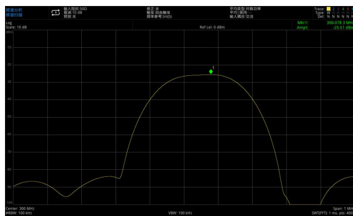
图 3-5：没有分辨出的两个等幅信号
