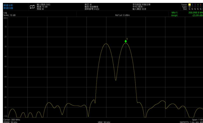
图 3-6：分辨出的两个等幅信号（1）
