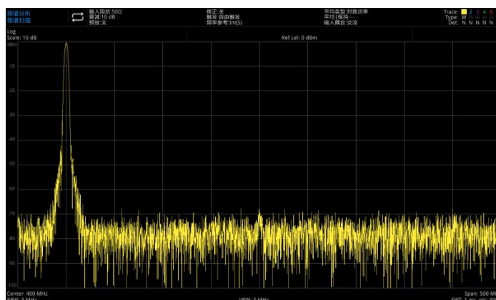
图 3-16 谐波失真
