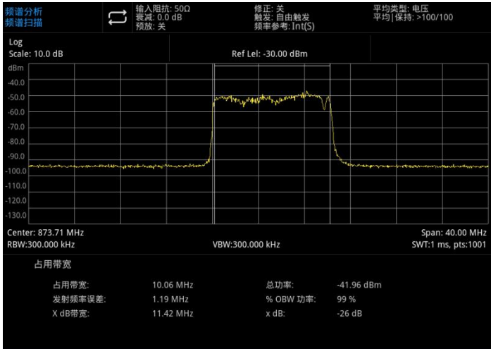
图 5-3：占用带宽
