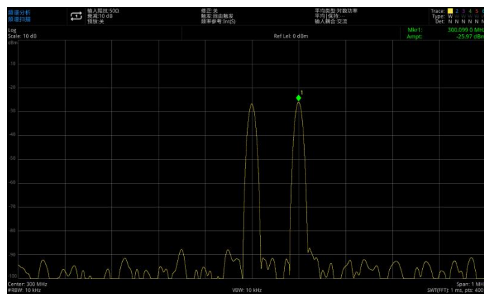
图 3-7: 分辨出的两个等幅信号 (2)
