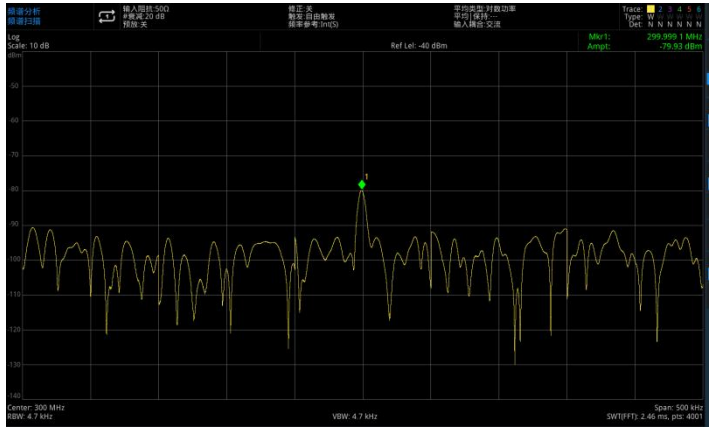
图 3-11：接近底噪的信号
