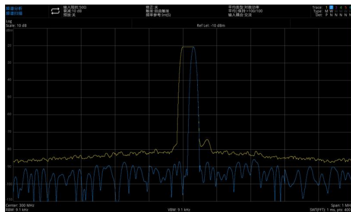
图 3-15：用最大保持和刷新来观察信号漂移
