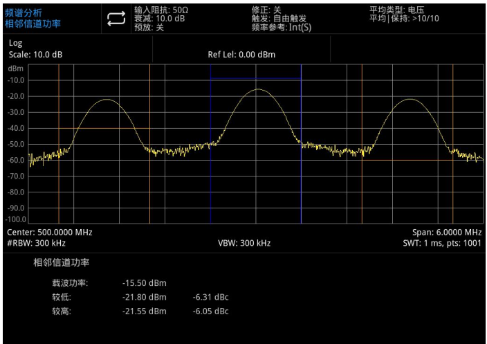
图 5-5：相邻信道功率测量
