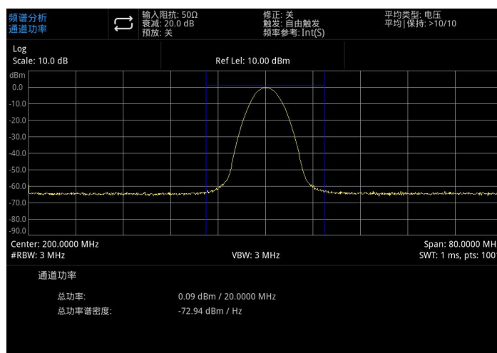
图 5-1: 通道功率
