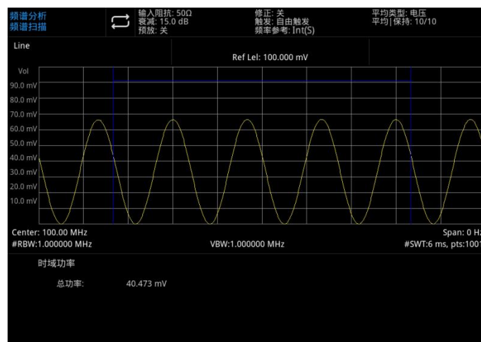
图 5-2：时域功率
