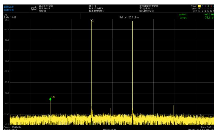
图 3-19：测量失真产物
