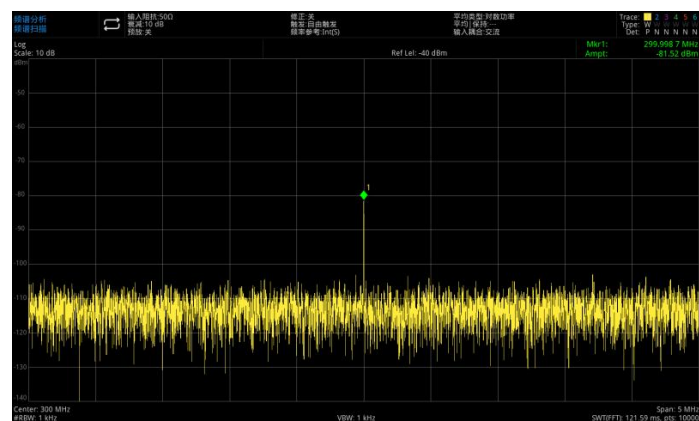
图 3-13: 减小分辨率带宽
