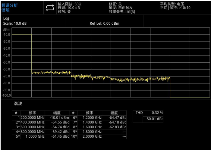
图 5-8：谐波测量
