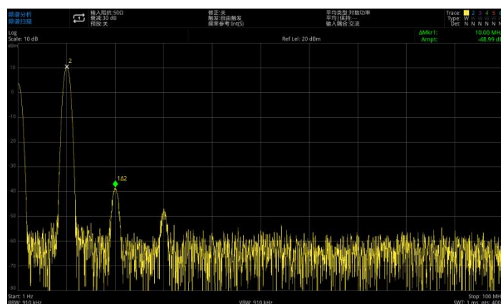
图 3-2：标记模式差值△在同一屏幕信号比较
