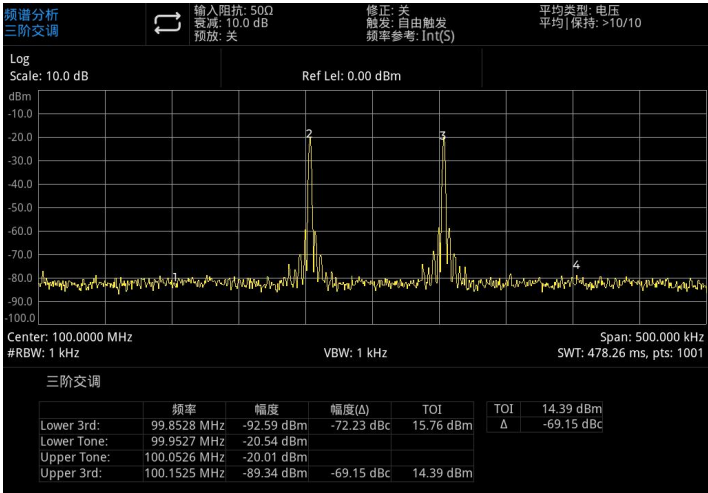
图 5-4：三阶交调
