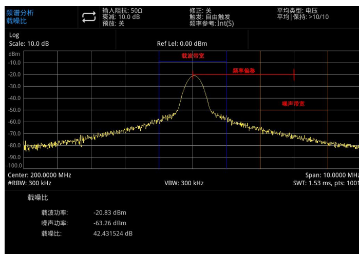
图 5-7：载噪比测量
