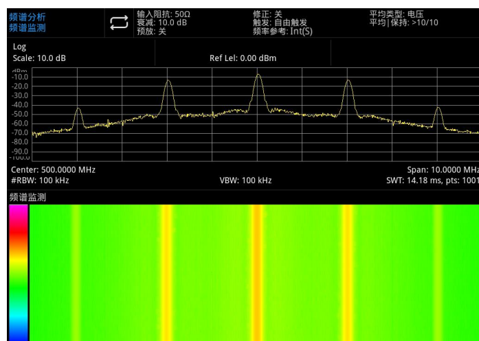
图 5-6：频谱监测
