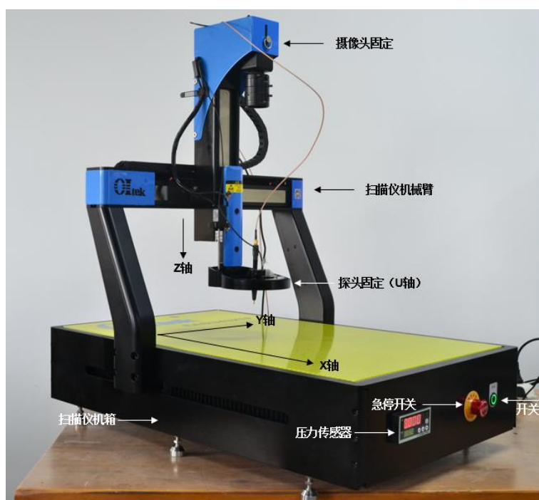
图 3 扫描仪组成
