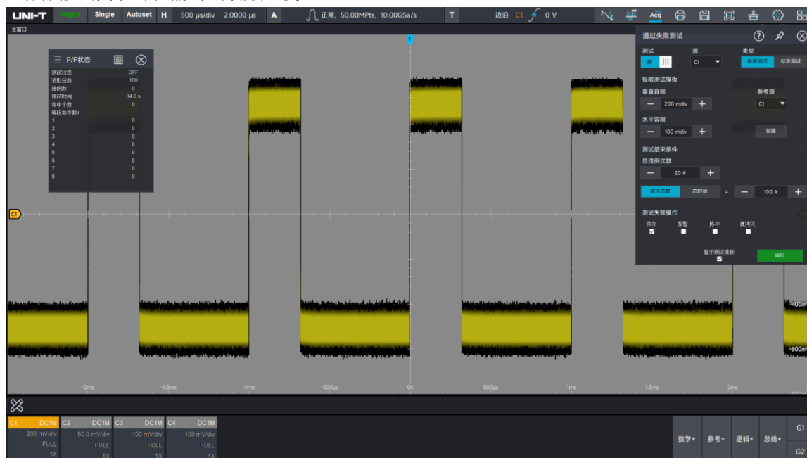
使用噪声最坏的极限创建测试模板，几秒即可完成符合标准的波形筛选
