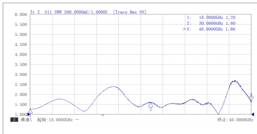
Input VSWR
