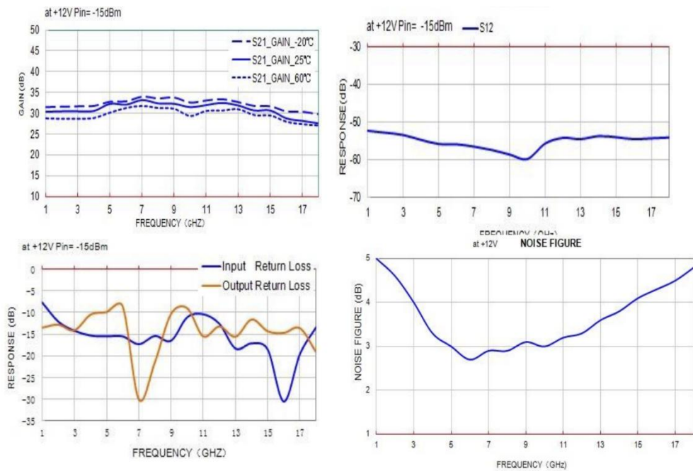
OI-AMP18G30 低噪声放大器特性
