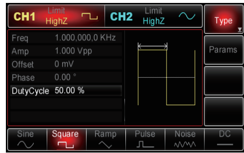
占空比为50%的方波信号
