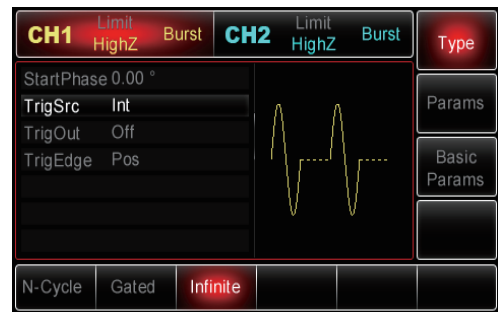
三种猝发模式
