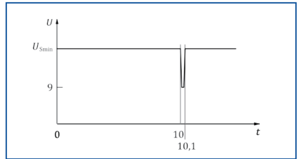
图8-24V电力系统短电压降
