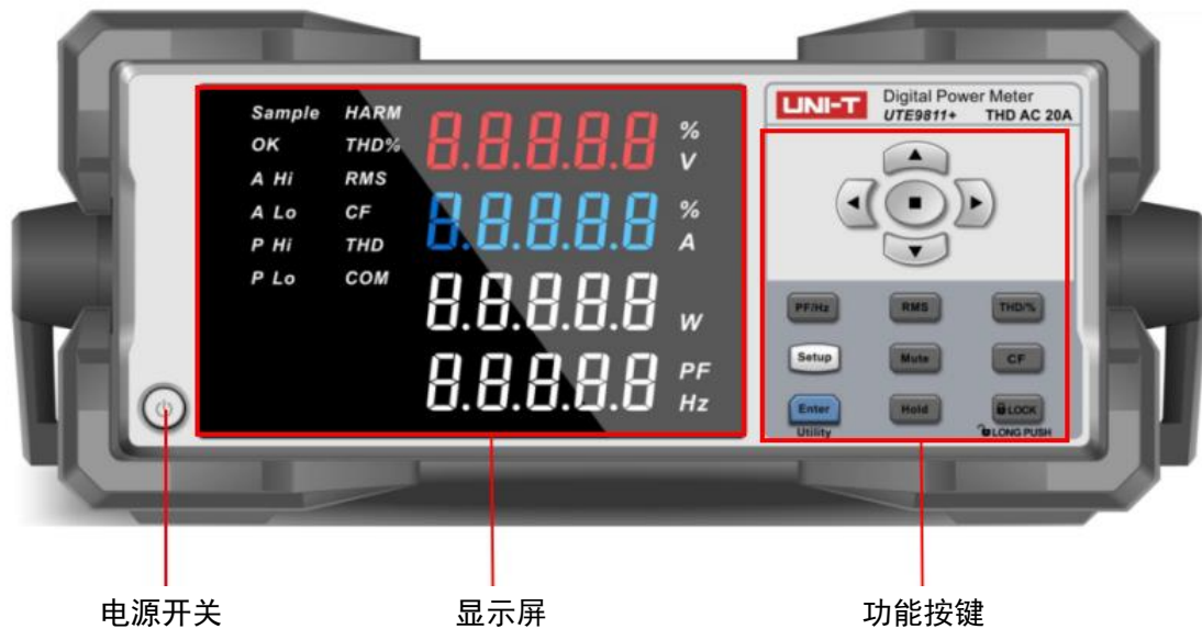
图 2.3.3 UTE11+前面板
