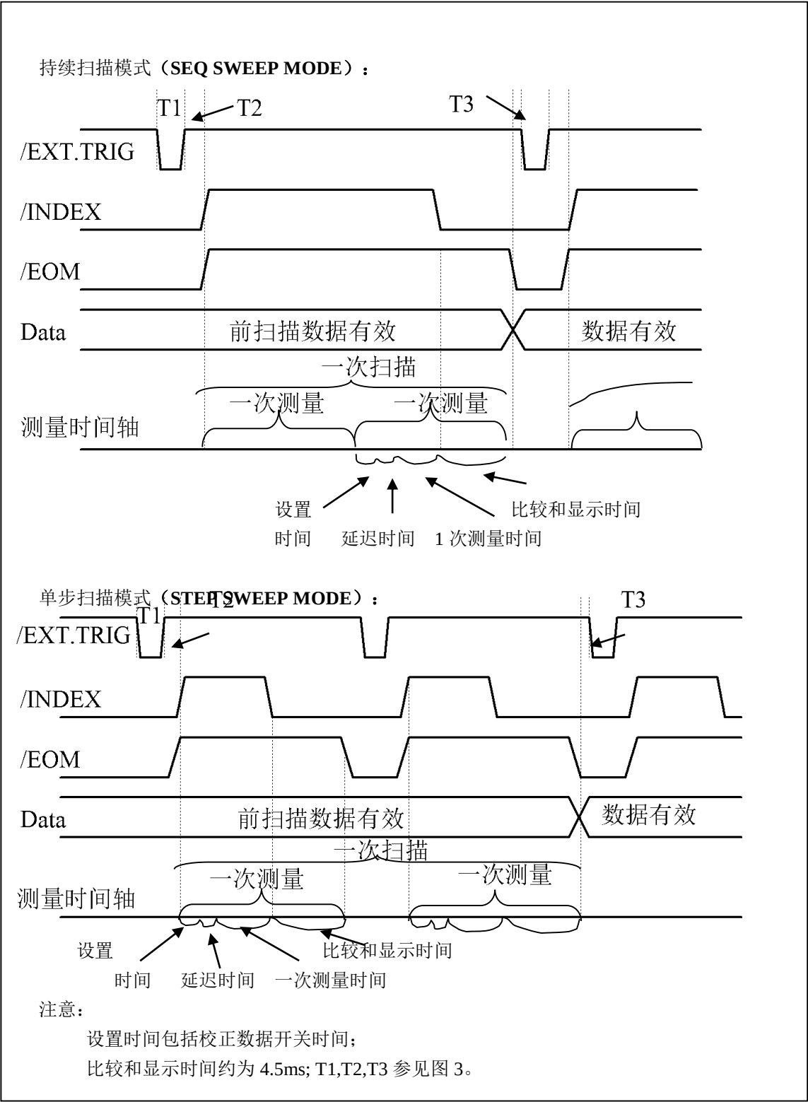
图 5 计时图解
