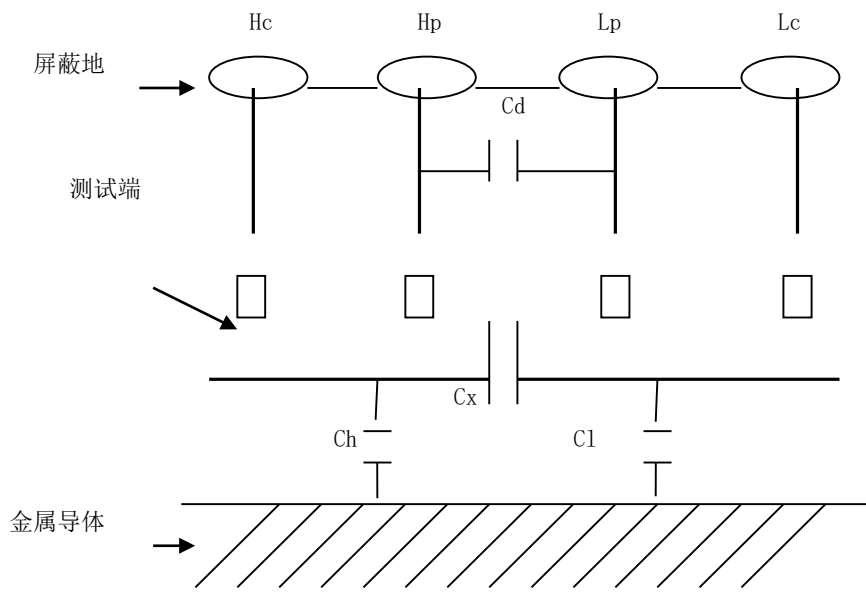
图 8-3-1 杂散电容的影响示意图
