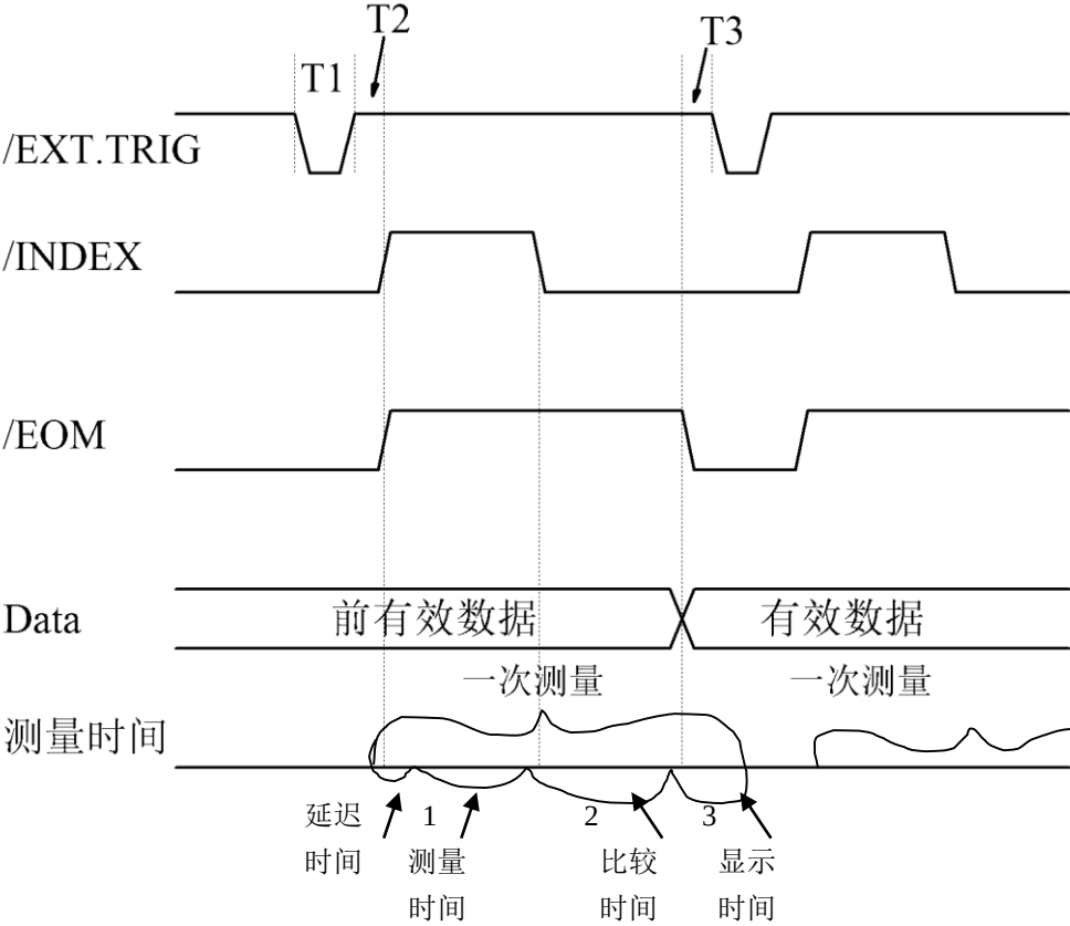
图 3 时序图
