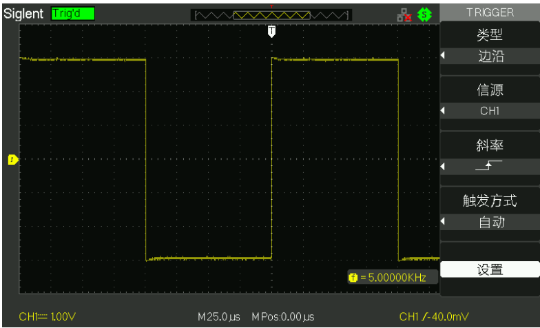
图 2-21 边沿触发
