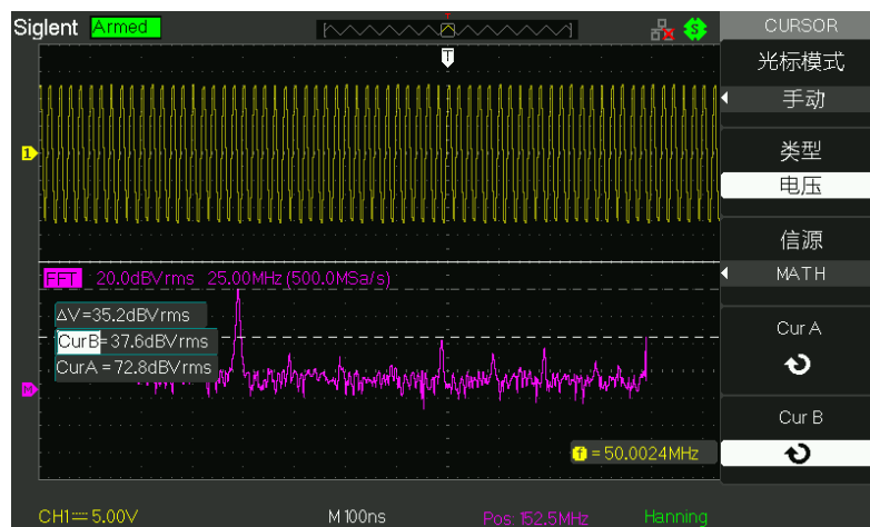
图 2-14 测定 FFT 谱幅度
