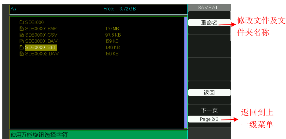
图 2-54 文件存储/调出菜单 3
