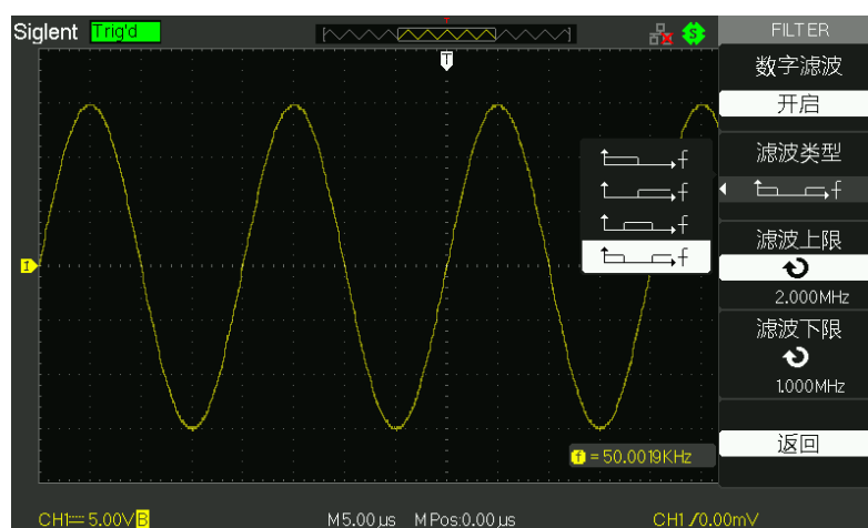
图 2-11 数字滤波设置
