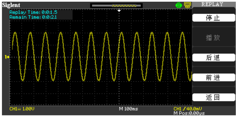
图 2-80 波形回放功
