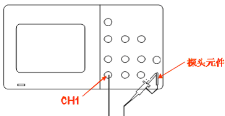
图 1-4 功能检查连接图
