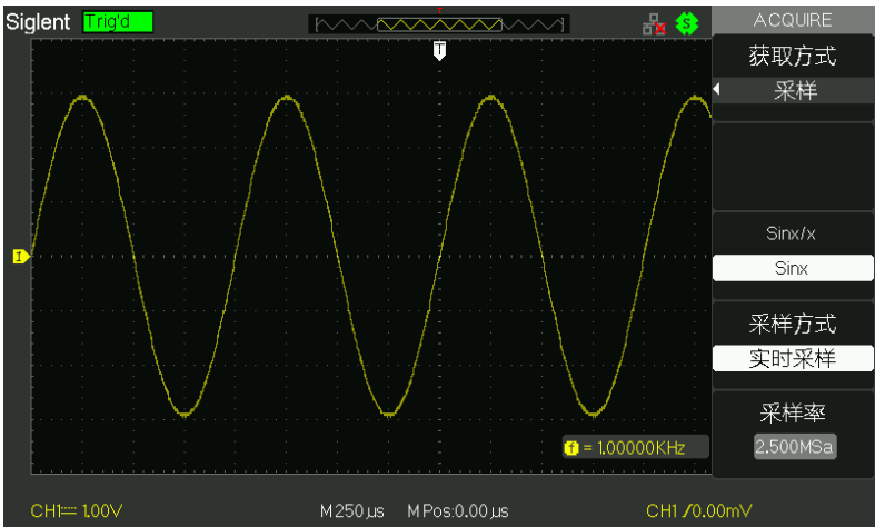
图 2-32 采样模式
