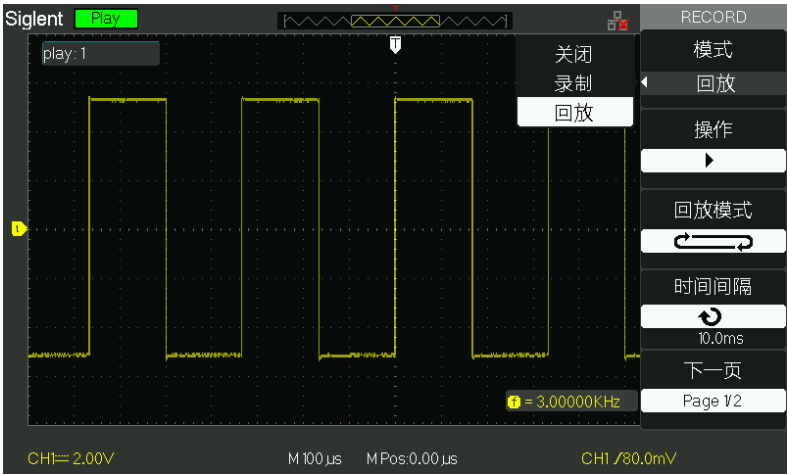
图 2-76 波形回放功能菜单 1
