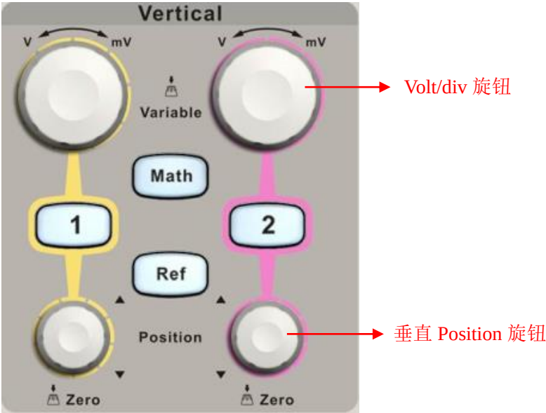
图 2-5 垂直系统
