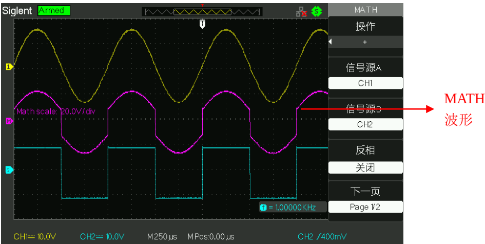
图 2-12 CH1 与 CH2 的波形相加
