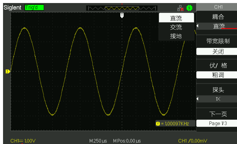
图 2-6 通道耦合设置
