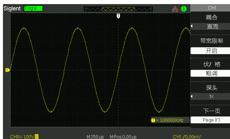
图 2-7 设置带宽限制
