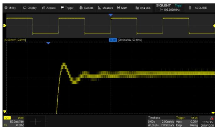
8-bit 模式
