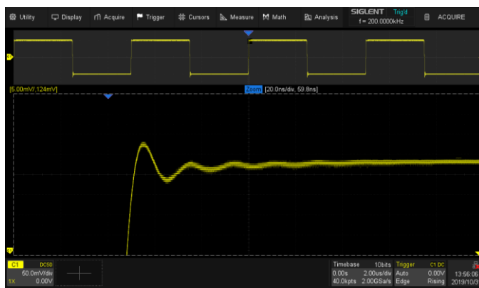
10-bit 模式
