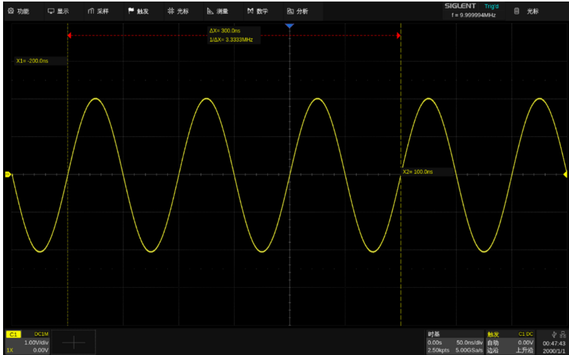
水平档位=50ns/div, X1= -200ns (-4div), X2= 100ns (2div)
