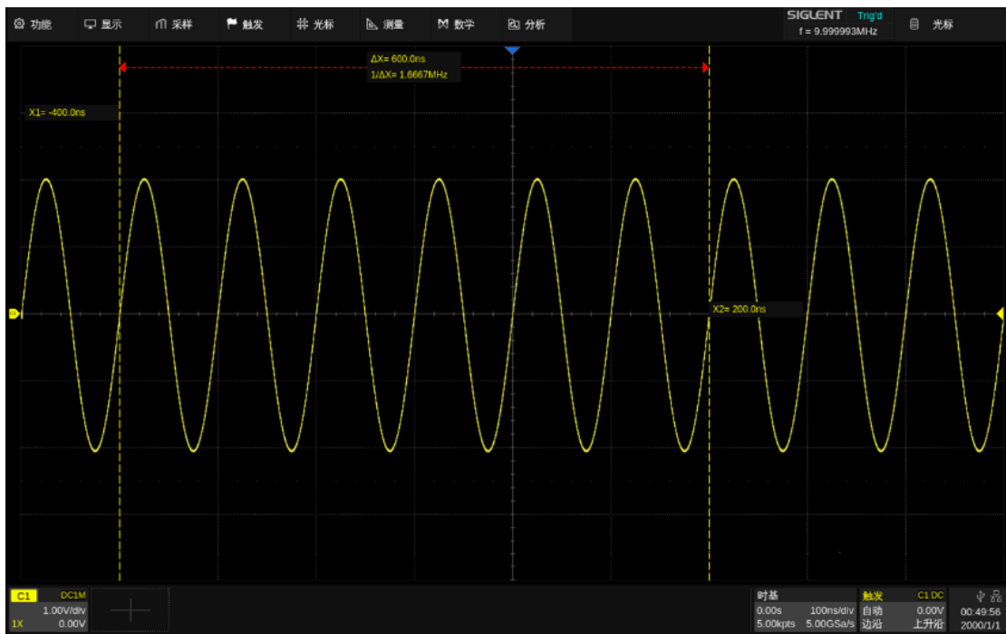
位置固定，水平档位设置为 100ns/div, X 光标的格数 (-4div、2div) 不变, X1、X2 数值变化为: -400ns、200ns
