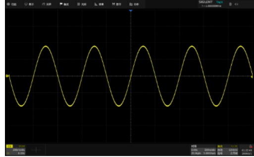
对话框关闭
