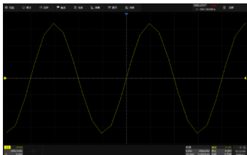
x 插值
