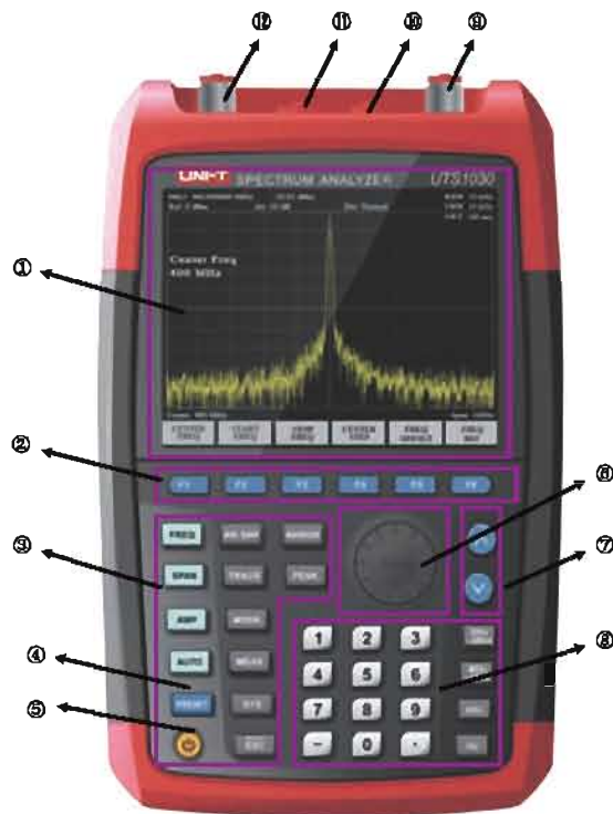
图 2-1 前面板视图
