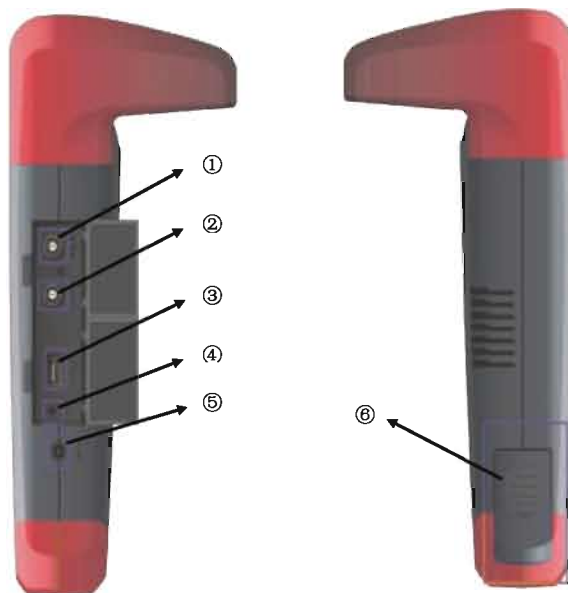
图 2-2 侧面板视图
