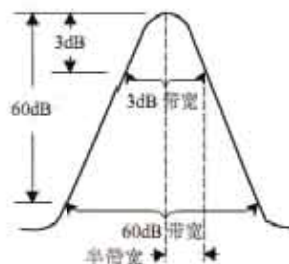
图4-4 带宽与矩形系数
