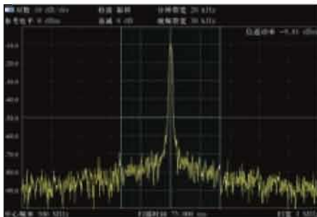
图4-10 信道功率测量结果
