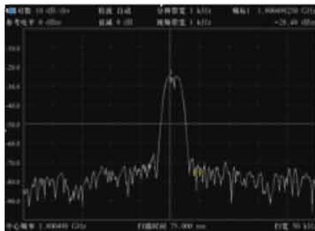
图4-2 1kHz分辨带宽
