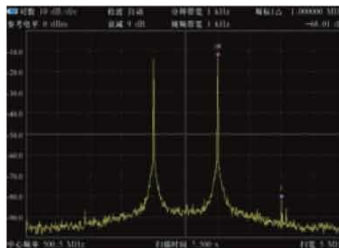
图4-14 三阶交调失真测量
