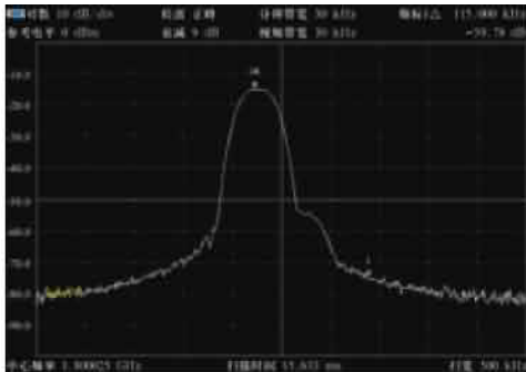
图4-5 30kHz 分辨带宽设置下的测试
