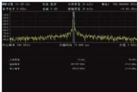
图4-11 占用带宽测量结果
