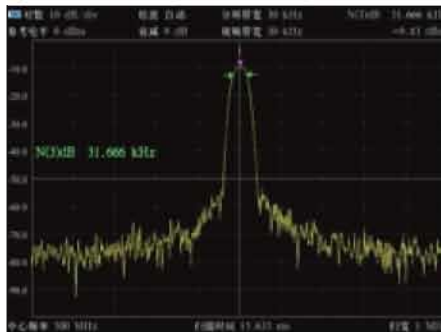
图4-8 N(3)dB带宽测量结果
