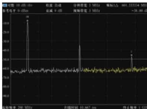
图4-13 谐波失真测量结果
