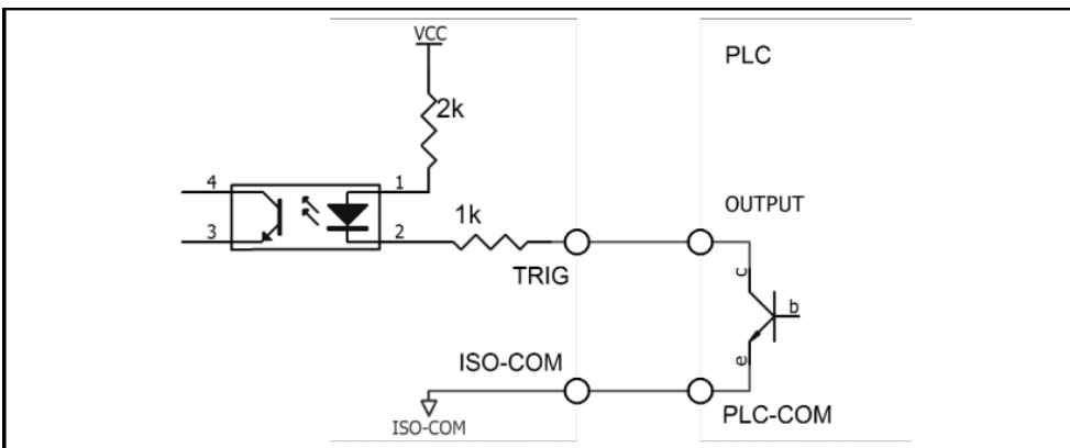
图 12-8 使用 PLC 负公共端子控制
