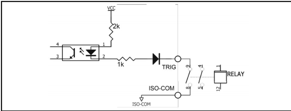
图 12-7 使用继电器控制
