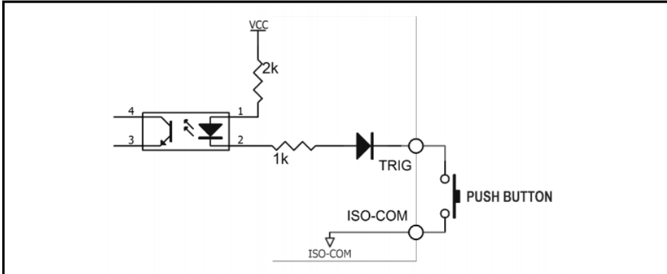
图 12-6 与开关的连接
