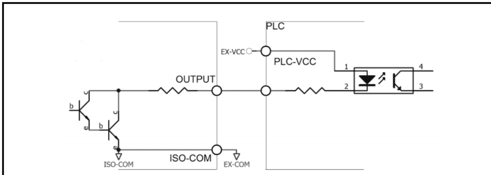
图 12-13 输出到 PLC 负公共端子
