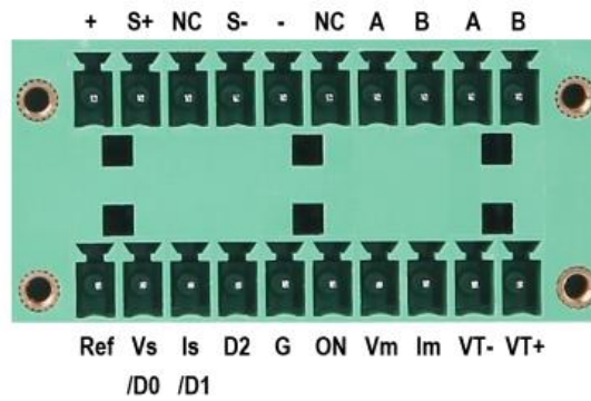
后面板端子图
