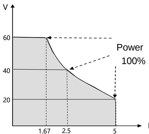
UDP6922B 输出I-V 曲线图
