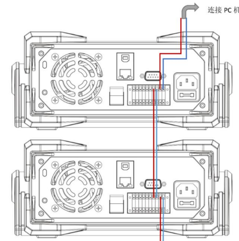
基于 RS485 多机通讯硬件连接
