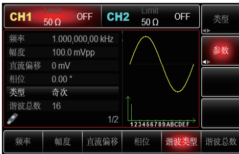
16次谐波输出
