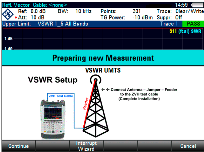
测试序列中的各单项测量可设置说明和图片以为用户提供有用信息
