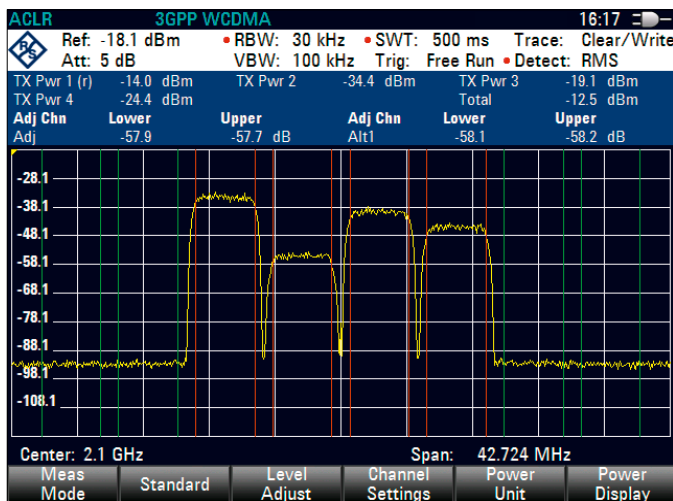
带四个载波的 3GPP WCDMA 信号的 ACLR 测量
