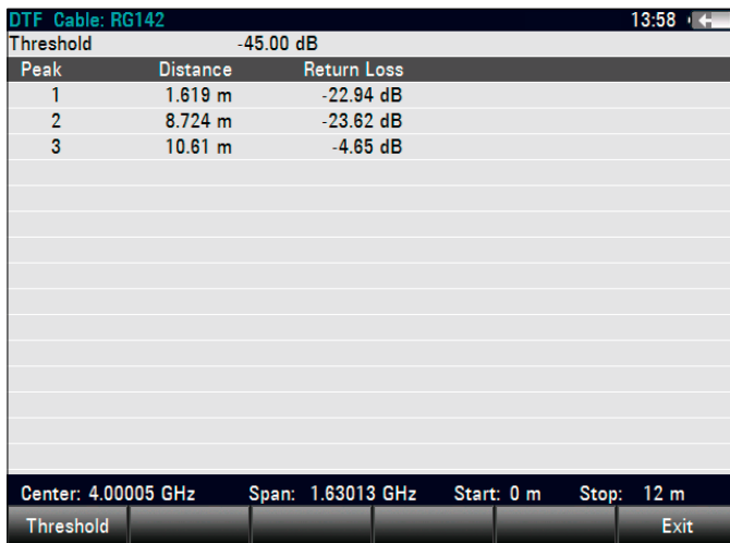
超出预定义阈值的电缆故障列表显示
