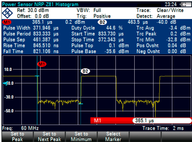
使用 R&S®ZVH-K29 和 R&S®NRP-Z81 宽带功率探头进行脉冲分析
