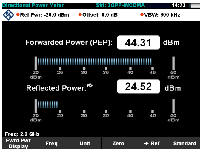
天线的前向功率（发射输出）和反射功率测量
