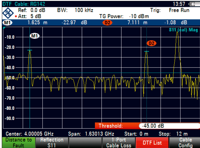
故障点距离 (DTF) 测量
