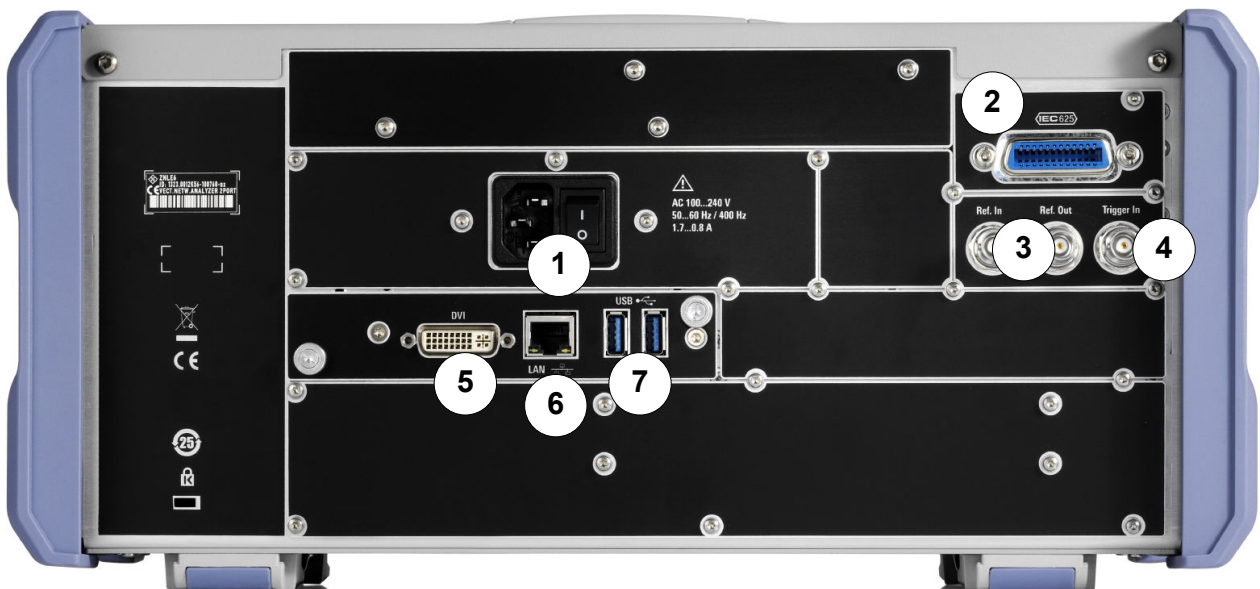
图 5-3: 后面板视图
