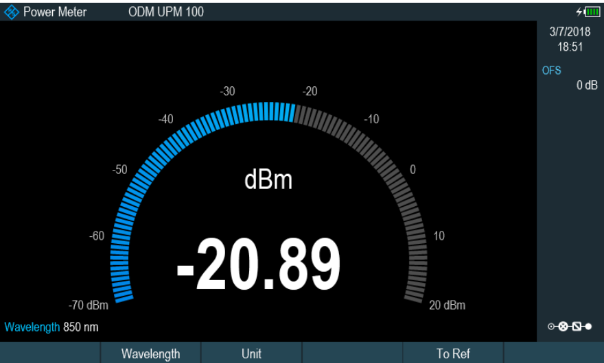
光功率测量屏幕 (R&S®FPH-K9)
