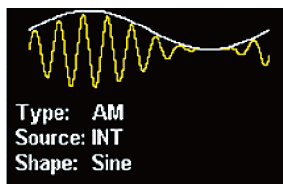
AM
