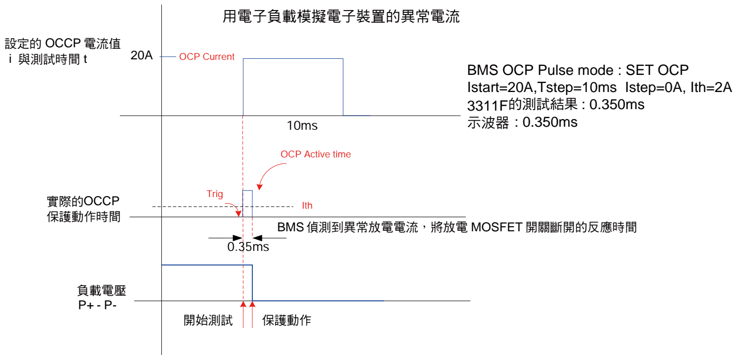
圖11 3311F的過放電流測試程序圖
