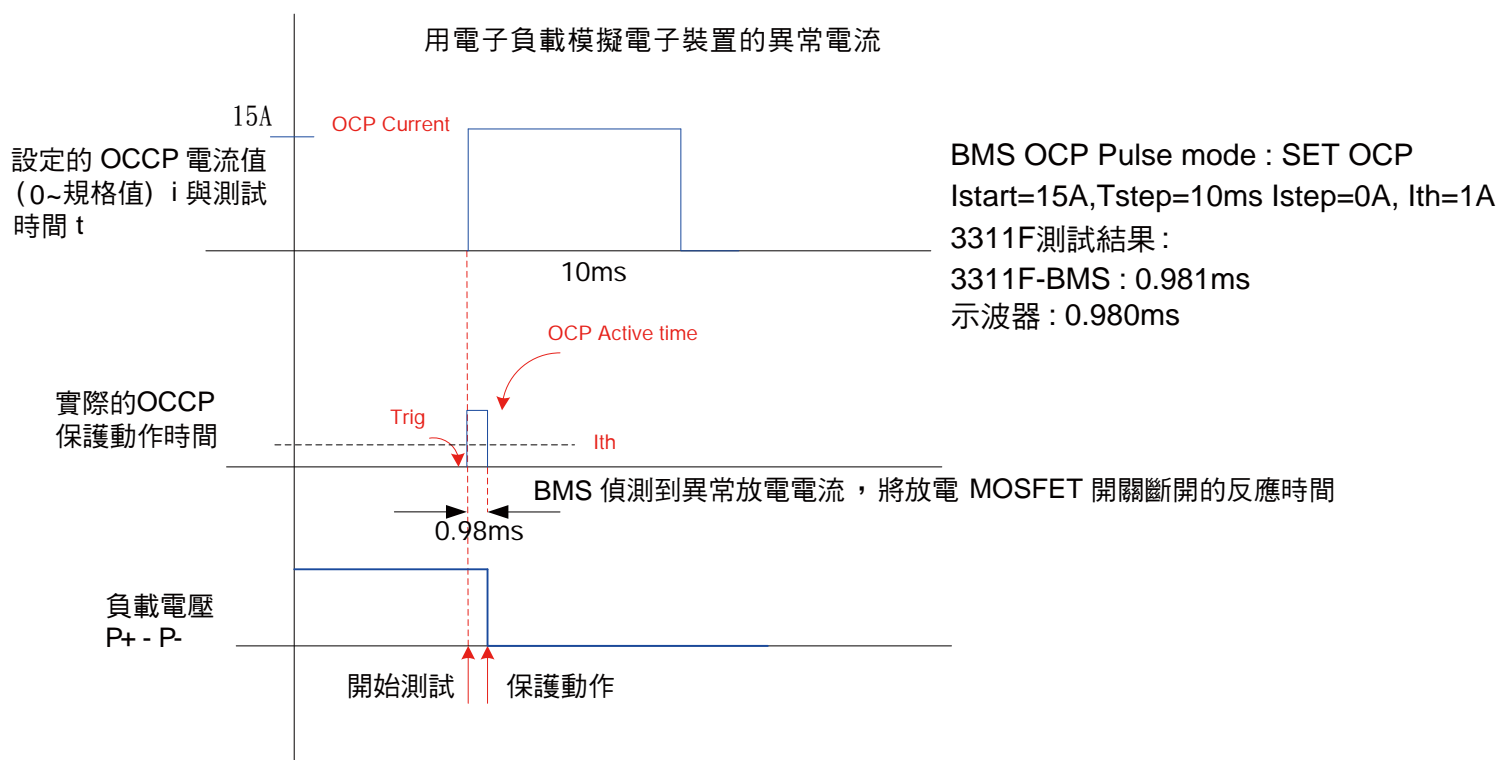
圖6 3311F的BMS過充電流測試程序圖 (單脈衝)
