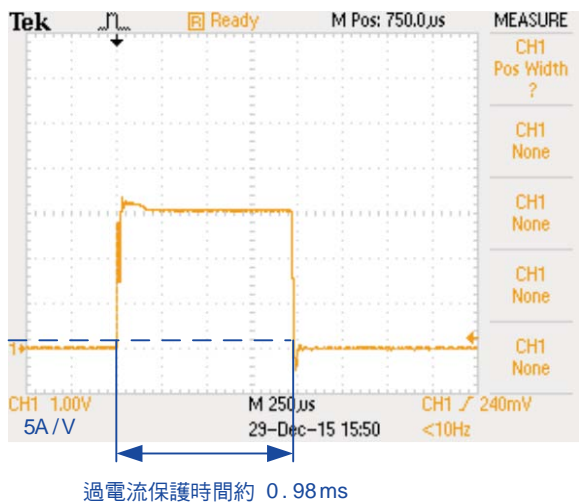
圖7 3311F的BMS過充電流測試結果 (單脈衝)
