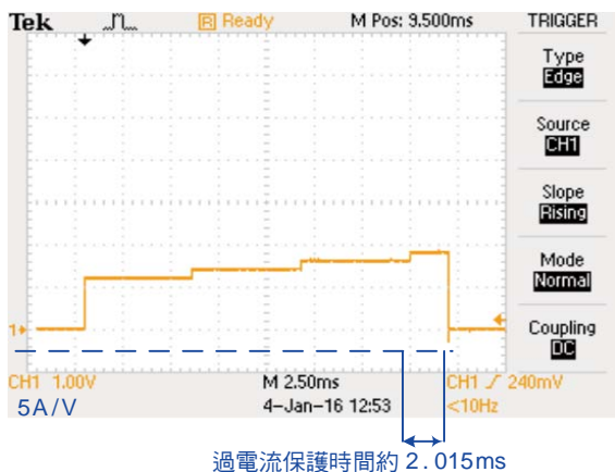
圖9 3311F的BMS過充電流測試結果(連續STEP脈衝)
