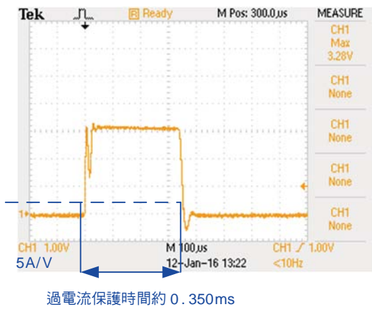
圖12 3311F的BMS過放電流測試結果(單脈衝)
