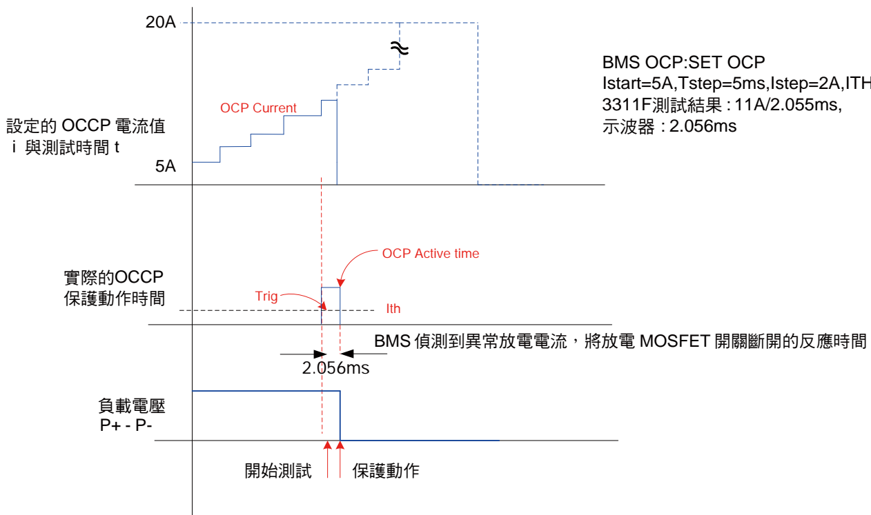
圖13 3311F的BMS過放電流測試程序圖(連續STEP脈衝)
