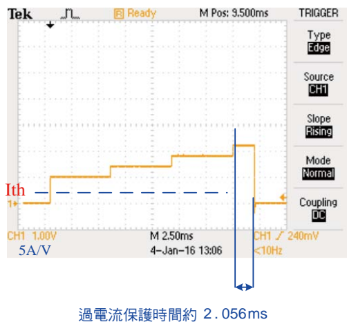
圖14 3311F的BMS過放電流測試結果(連續STEP脈衝)
