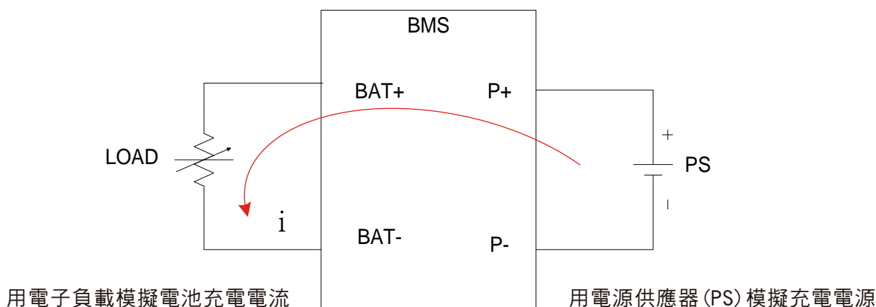
圖5 BMS充電時的等效模擬圖
