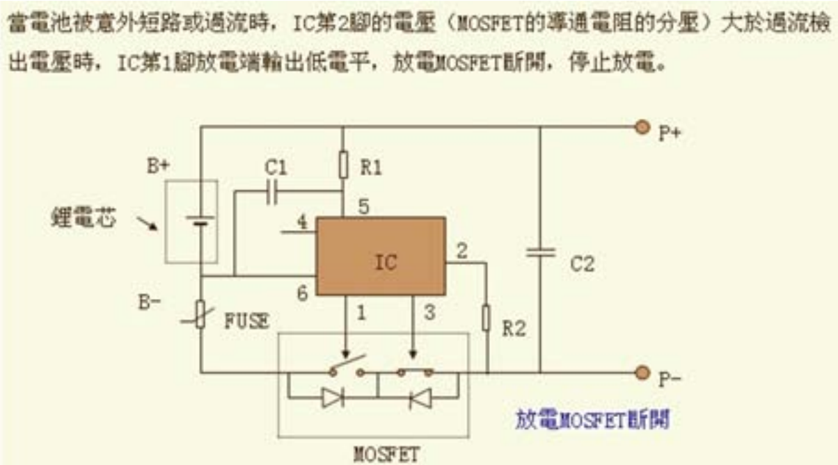
圖1 BMS 的內部架構
