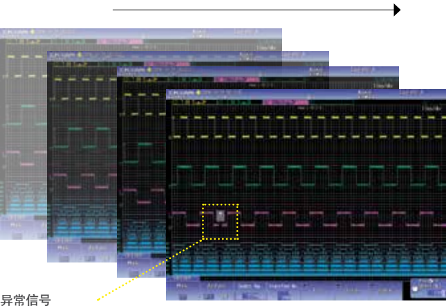
历史波形
