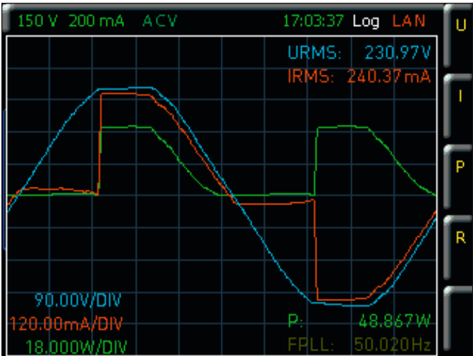
波形功能: 带有相位角控制的负载
