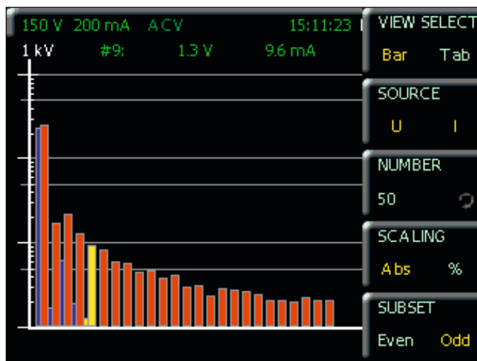
谐波分析: 条棒
