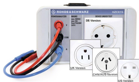
不同国家的插头型式（含中国）：OIHZC815-CHN
