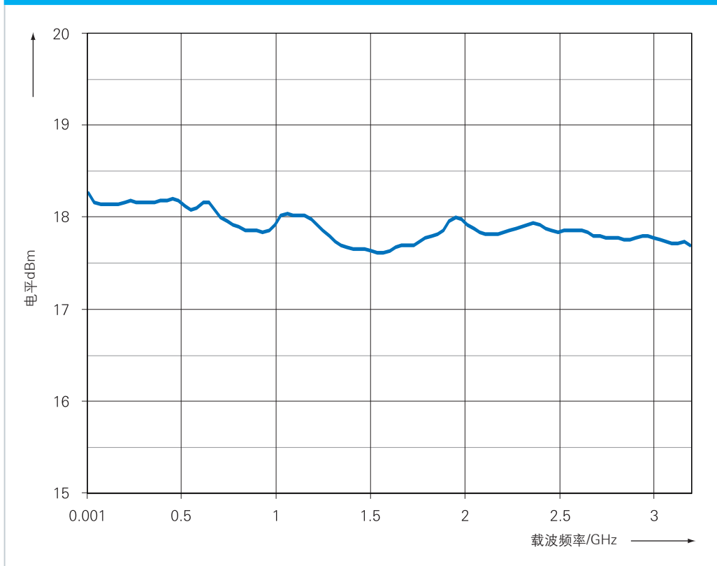
所测得的最大可用输出功率
