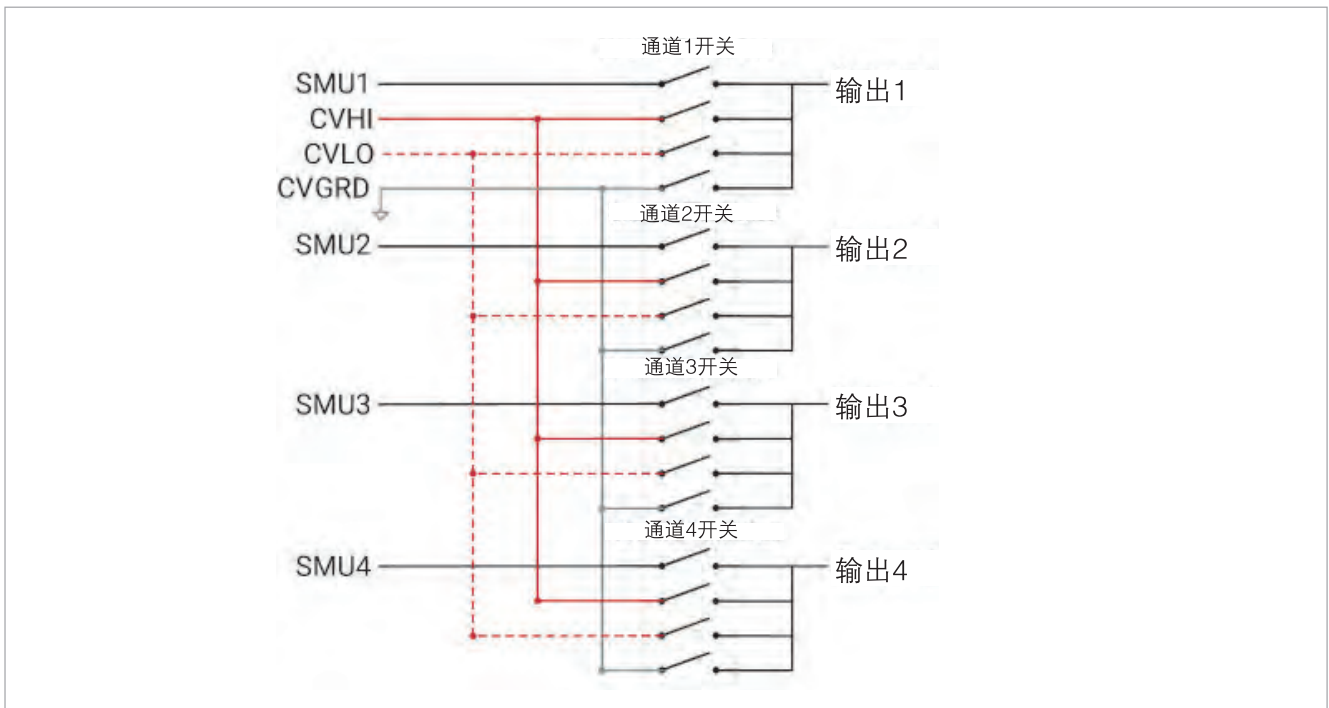
4200A-CVIV 多通道开关连接示意图。
