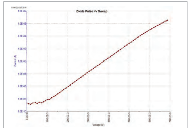
4225-RPM 为脉冲应用提供了更低的电流范围。
