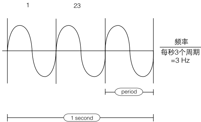
图 8. 正弦波的频率和周期。
