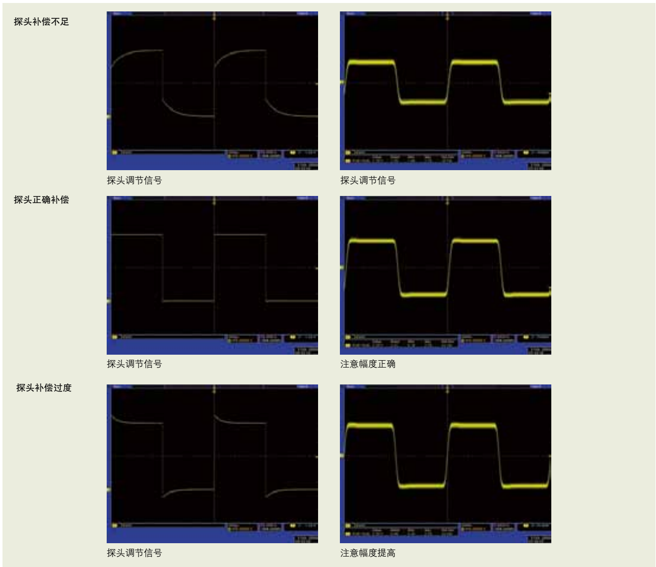
图 65. 探头补偿不当的影响。
