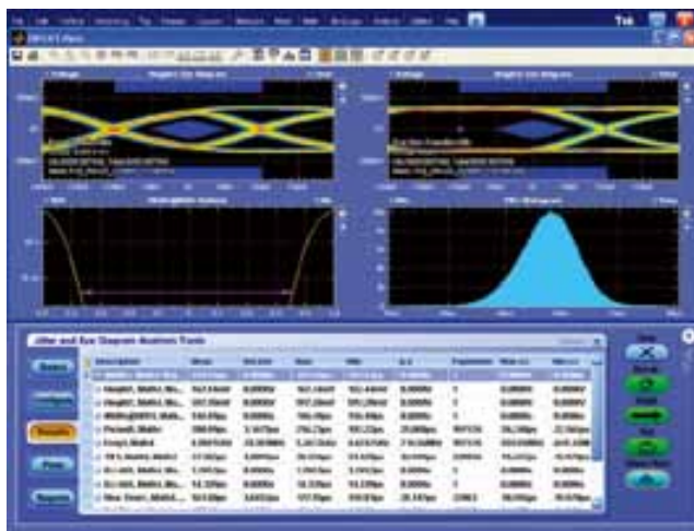
图 54. 分析软件包是为满足当前高速数字设计人员的抖动和眼图测量需求专门设计的。
