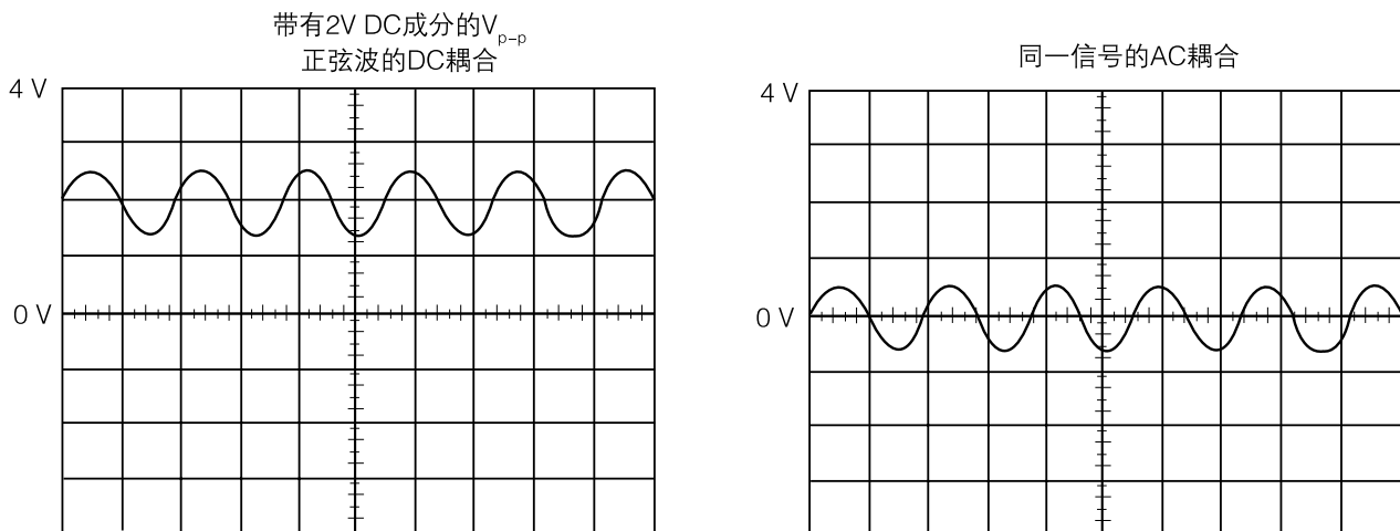
图 21. AC 和 DC 输入耦合。
