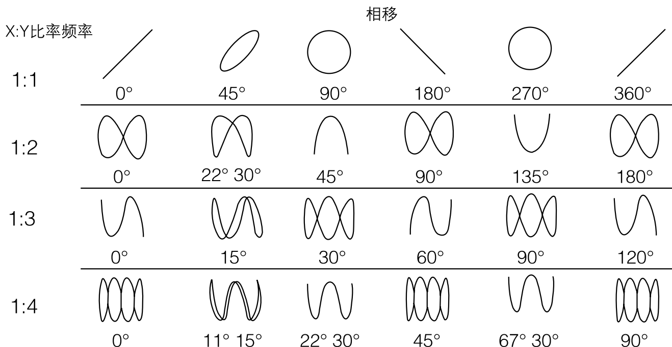
图 70. Lissajous 码型。
