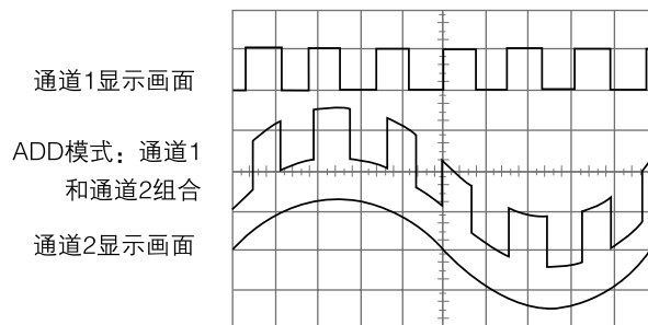
图 38. 增加通道。
