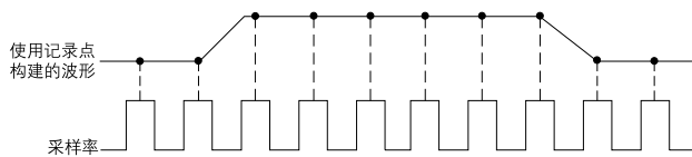
图 26. 实时采样方法。
