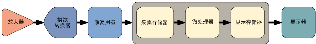
图 12. 数字存储示波器 (DSO) 的串行处理结构。
