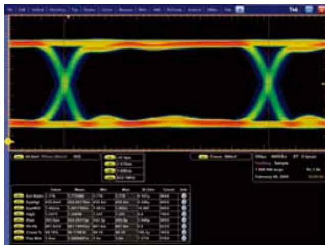
图 7. 622 Mb/s 串行数据眼图。
