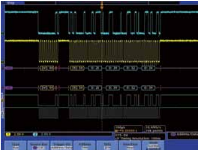
图 55. 自动触发、解码和搜索串行数据包上下文加快了串行总线分析速度。
