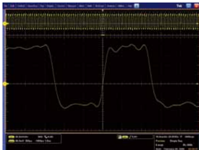
图 46. 检定高速数字信号的上升时间。
