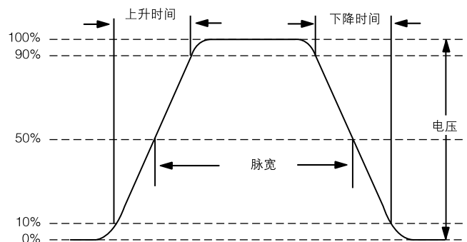
图 69. 上升时间和脉宽测量点。
