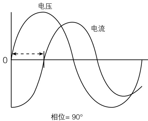
图 10. 相移。
