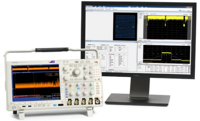
MDO4000B 与 SignalVu-PC 配套使用以分析 802.11ac 调制。
