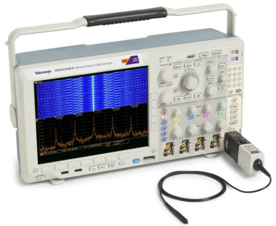
选配的 TPA-N-VPI 适配器可以把任何有源 50 Ω TekVPI 探头连接到频谱分析仪上。
