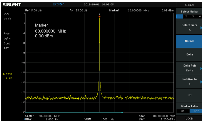
◀ 高保真正弦波输出，在 60MHz, 0dBm 时几乎观测不到非谐波杂散
