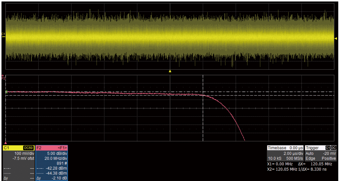
▲ 输出白噪声测试获得的系统 -3dB 带宽在 120MHz 以上
