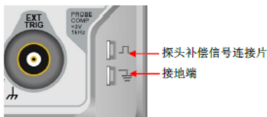
图 4-1 探头补偿信号连接片和接地端
