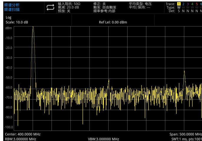
图 3-16 谐波失真
