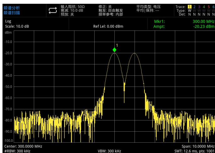
图 3-6: 分辨出的两个等幅信号 (1)
