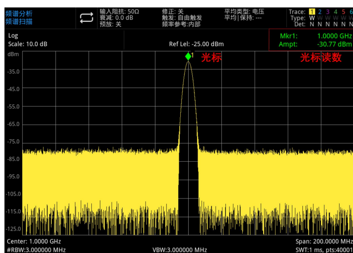
图 4-1：标记光标读数
