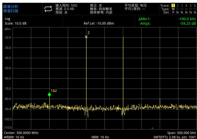
图 3-19: 测量失真产物
