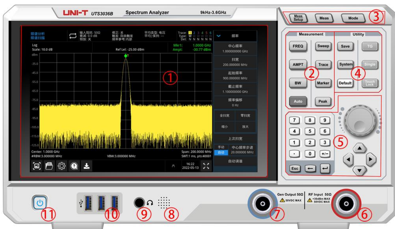
图 1-1: 前面板
