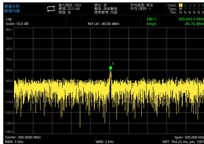
图 3-11: 接近底噪的信号
