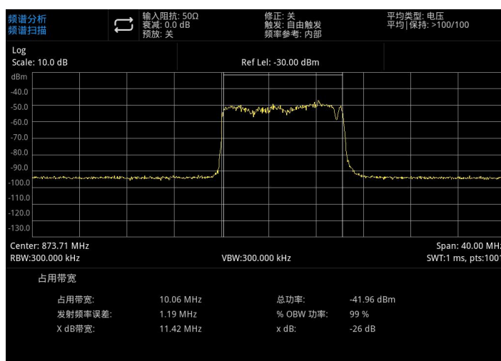
图 5-3:占用带宽
