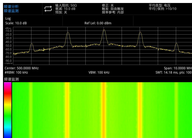
图 5-6：频谱监测
