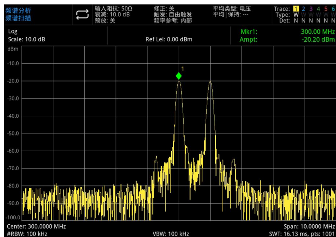
图 3-7: 分辨出的两个等幅信号 (2)
