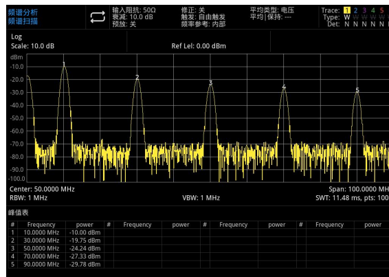
图 4-3：峰值表
