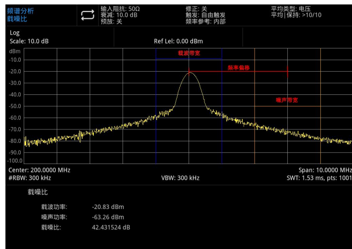
图 5-7：载噪比测量
