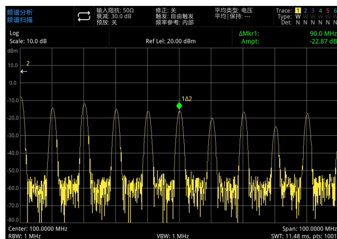
图 3-3：参考信号在屏幕外的 Delta 标记
