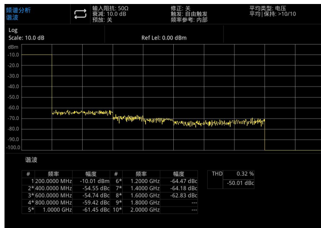
图 5-8: 谐波测量
