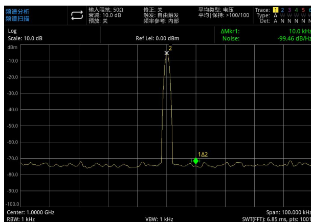
图 3-20: 相位噪声
