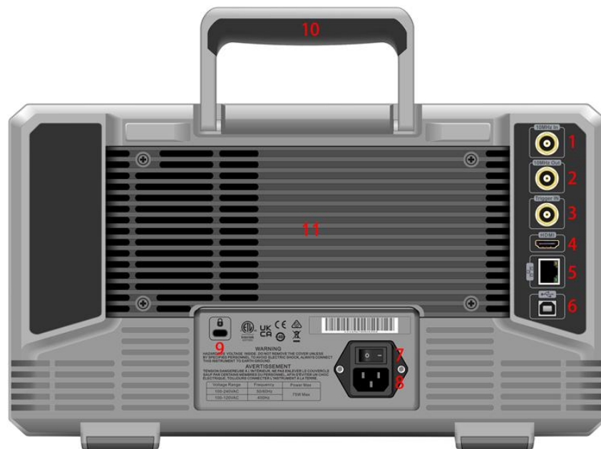
图 1-3: 后面板
