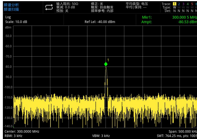
图:3-12: 在 0dB 衰减下测量小信号
