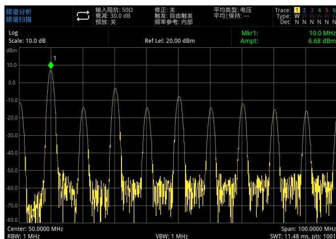
图 3-1：读出频率幅度
