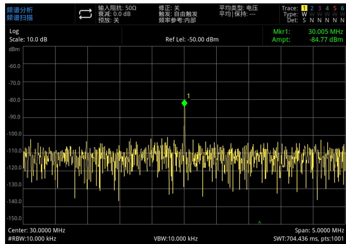
图 3-13: 减小分辨率带宽
