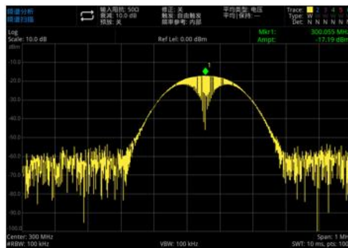
图 3-5: 没有分辨出的两个等幅信号
