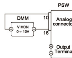
外部DMM监控输出电压
