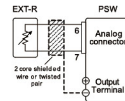
外部电阻控制电压输出
