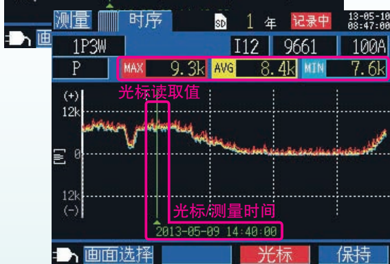
以5分钟为间隔图表显示24小时的测量值
