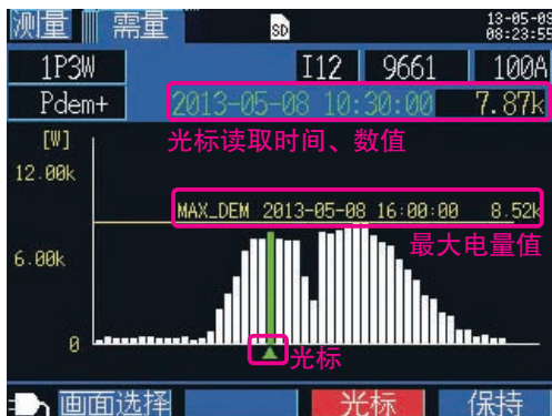
以30分钟为间隔柱状图显示24小时的测量值
