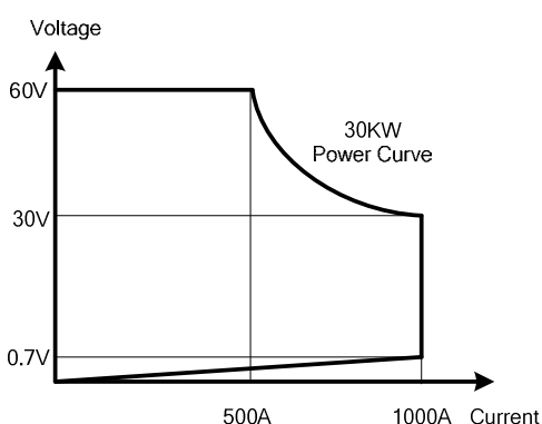
1-1.6 34130高功率電子負載功率曲線圖
