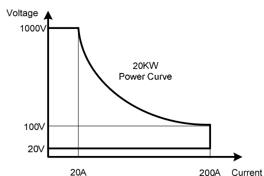
1-1.16 34320高功率電子負載功率曲線圖
