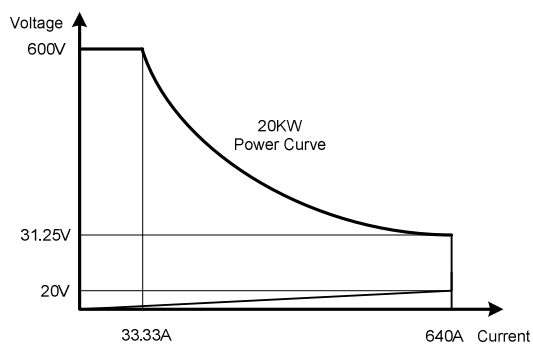
1-1.10 34220高功率電子負載功率曲線圖
