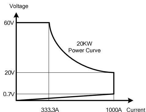
1-1.4 34120高功率電子負載功率曲線圖
