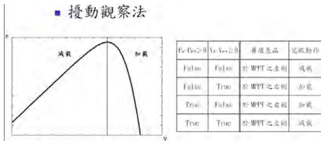
圖 5-12 擾動觀察法動作方式
