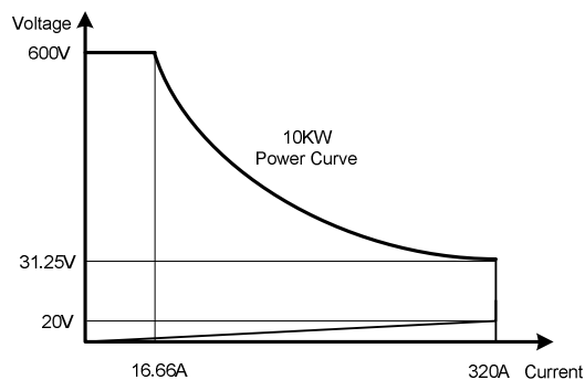
1-1.8 34210高功率電子負載功率曲線圖
