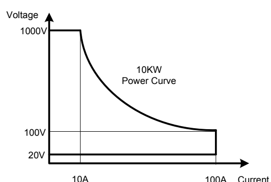
1-1.14 34310高功率電子負載功率曲線圖
