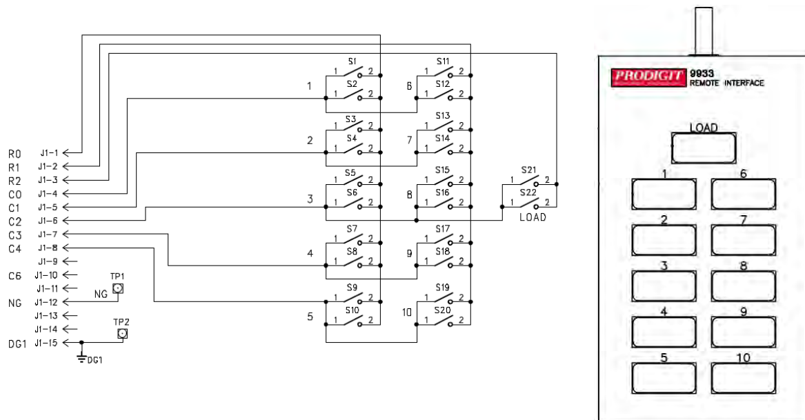
圖 2-9 9933 遙控器連接埠圖
