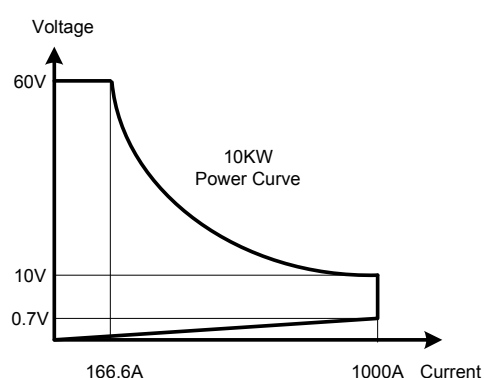
1-1.2 34110高功率電子負載功率曲線圖
