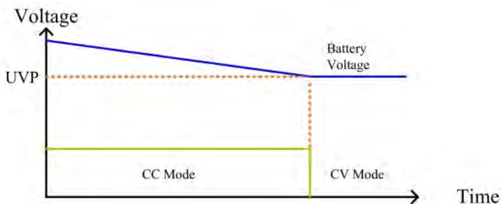
圖 5-14 電池放電測試-TYPE2
