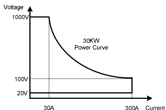
1-1.18 34330高功率電子負載功率曲線圖
