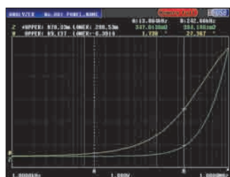
频率扫描测量 Z- \theta 测量画面
