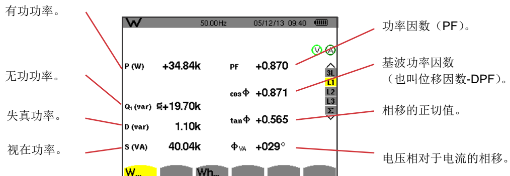
图 101: L1功率及相关量的显示页面
