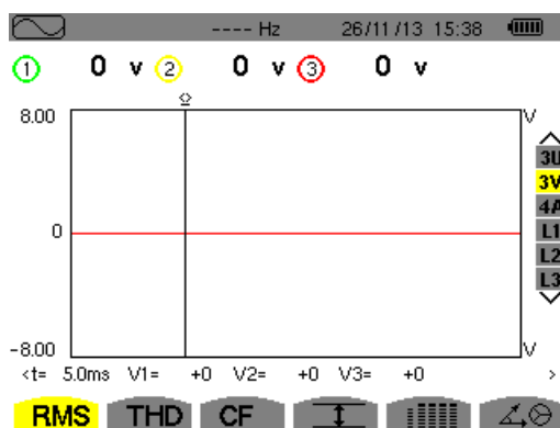
图 91: 波形图屏幕
