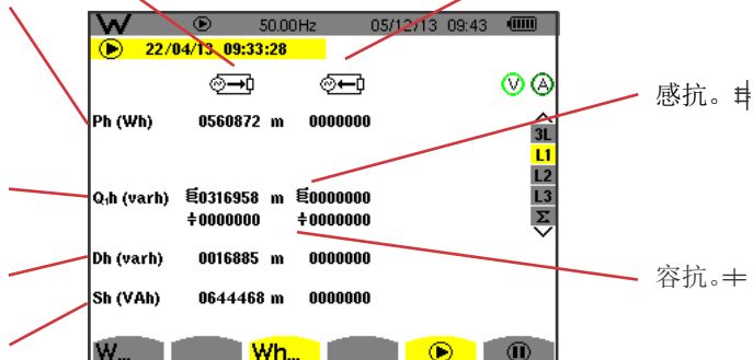
图 102: L1 电能消耗及生成显示页面
