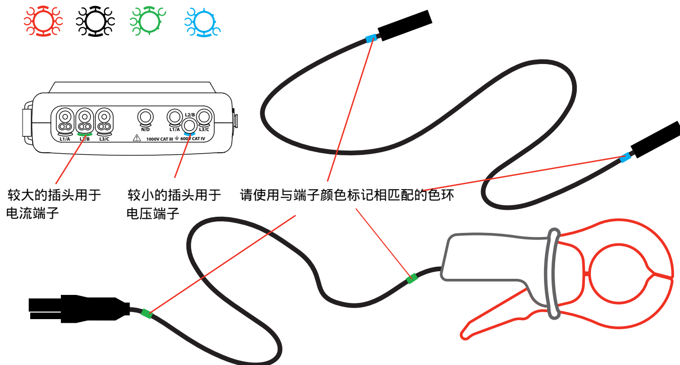
图10：导线及端子识别
