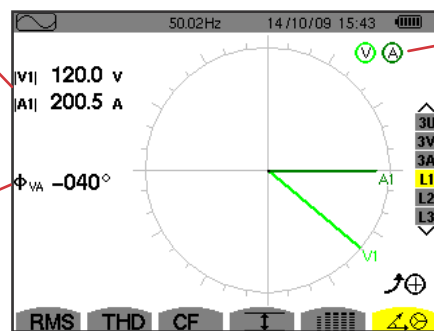
图 72: L1 菲涅尔图显示页面
