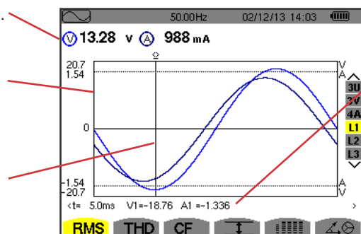
图 56: L1 RMS显示页面
