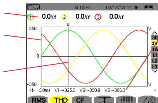
图 58: 3V THD显示页面
