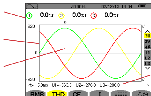
图 57: 3U THD显示页面
