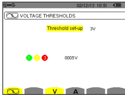
图29: 暂态模式设置菜单中的电压阈值设置页面
