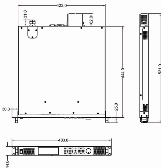
1U电源
